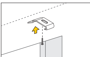
Halter an die Decke | in die Nische montieren. Nischenmaß ist 1 cm größer als das Anlagenmaß
