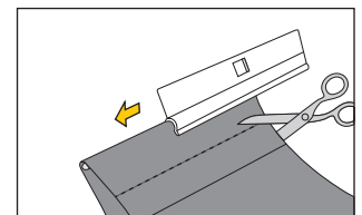
Lamellenhalter vorsichtig aufschieben. Überstehenden Stoff mit Schere entfernen
